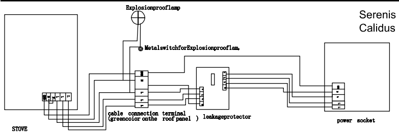
380v wiring diagram LM-T03B LM-T03A 380 V-nál min 20-25 A-es biztosíték kell
