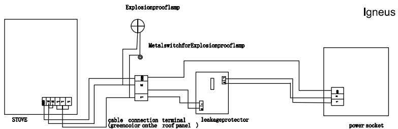
230 V-nál min 20A-es biztosíték kell 230v wiring diagram LM-T02B
