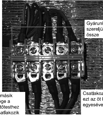
5-vezeték kábel
